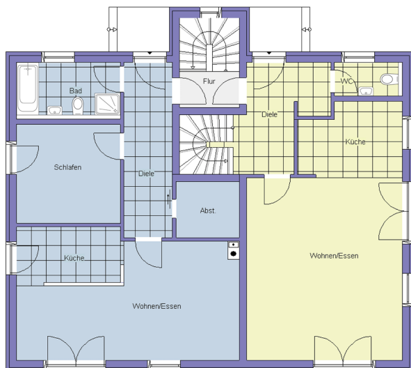
Erdgeschoss
