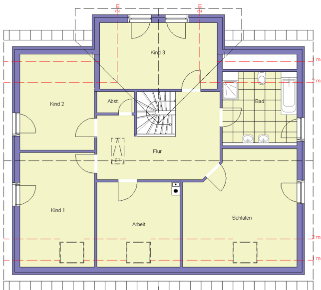
Dachgeschoss
